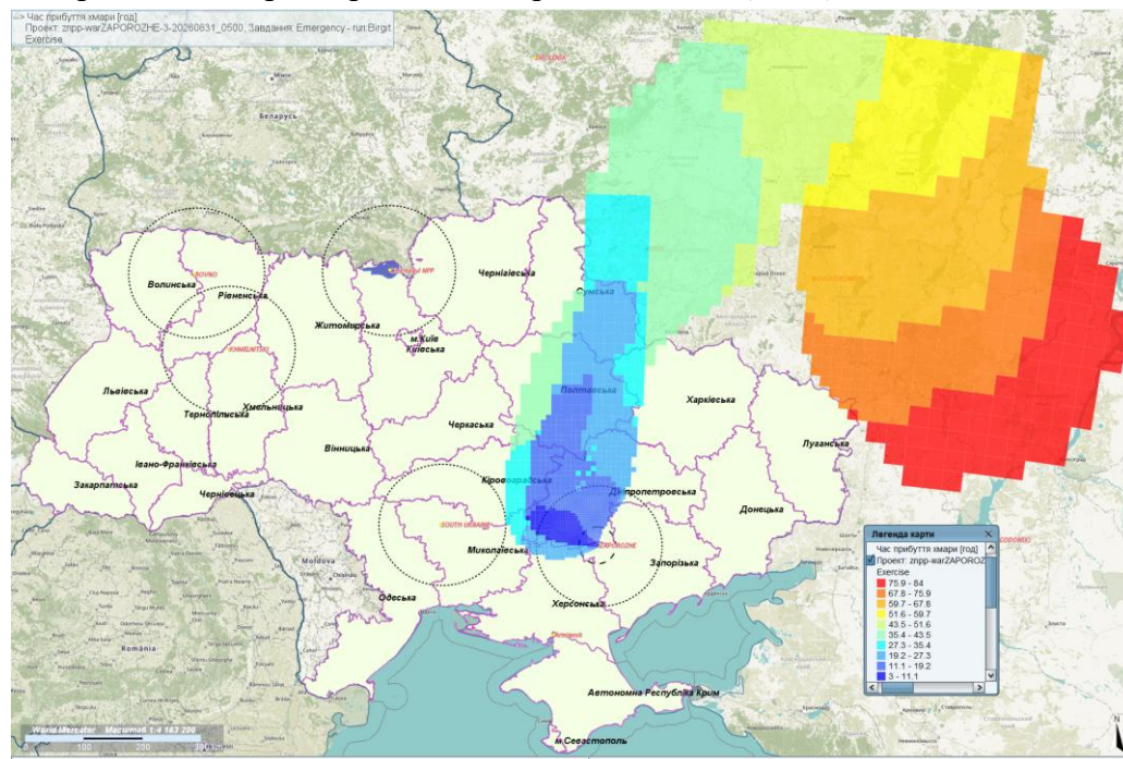
Рис.2. Прогноз поширення атмосферних мас з викидами ЗАЕС як наслідок УРА за 84 години. Час прибуття хмари. Швидкість поширення забруднення у годинах. Розрахунок умовного викиду з 08:30 (Київ) 31/08/2026. Тривалість умовного викиду 24 год.
