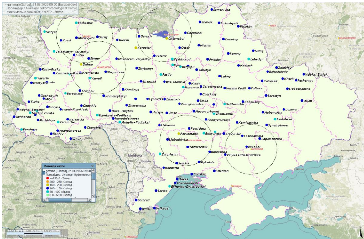
Рис1. Потужність дози Гамма-випромінювання на території України за результатами спостережень мережі НГМС станом на 09:00 (Київ) 31/08/2026.
