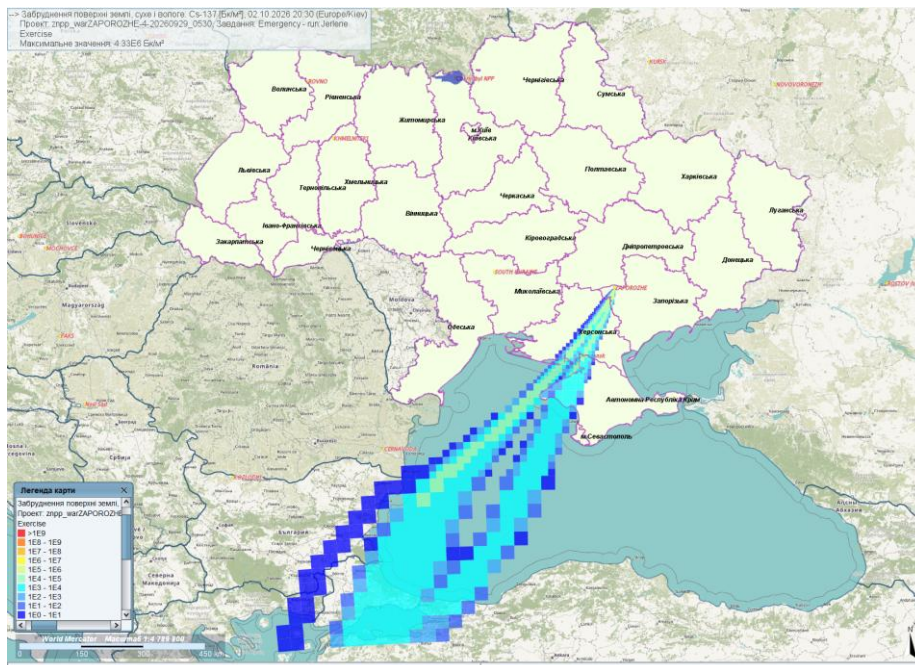
Рис.3. Результат моделювання просторового розподілу наслідків УРА на ЗАЕС (структура поля випадінь довгоіснуючих радіоактивних елементів на прикладі Цезію-137, згідно з НРБУ-97 таб. Д.8.1.). Щільність випадінь представлено у Бк/м². Розрахунок умовного викиду ЗАЕС з 8:30 (Київ) 29/09/2026
