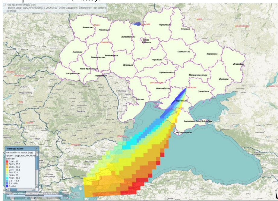
Рис.2. Прогноз поширення атмосферних мас з викидами ЗАЕС як наслідок УРА за 37 годин. Час прибуття хмари. Швидкість поширення забруднення у годинах. Розрахунок умовного викиду з 8:30 (Київ) 29/09/2026. Тривалість умовного викиду 24 год.
