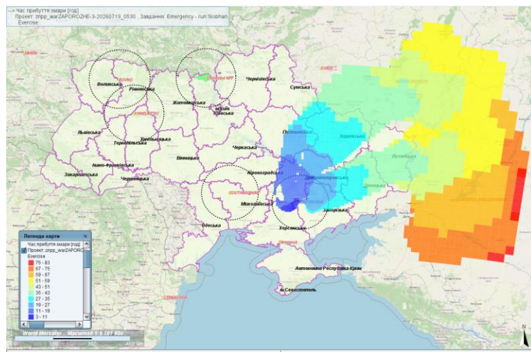
Рис.2. Прогноз поширення атмосферних мас з викидами ЗАЕС як наслідок УРА за 83 години. Час прибуття хмари. Швидкість поширення забруднення у годинах. Розрахунок умовного викиду з 09:00 (Київ) 19/07/2026. Тривалість умовного викиду 24 год.
