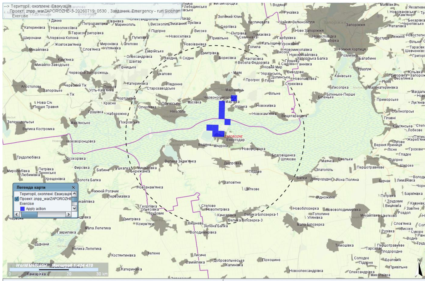
Рис.4. Результат моделювання просторового розподілу наслідків УРА на ЗАЕС (території, на яких рекомендована евакуація, згідно з НРБУ-97 таб. Д.8.1.). Пунктиром позначено 30-ти кілометрову зону ЗАЕС. Розрахунок умовного викиду ЗАЕС з 09:00 (Київ) 19/07/2026
