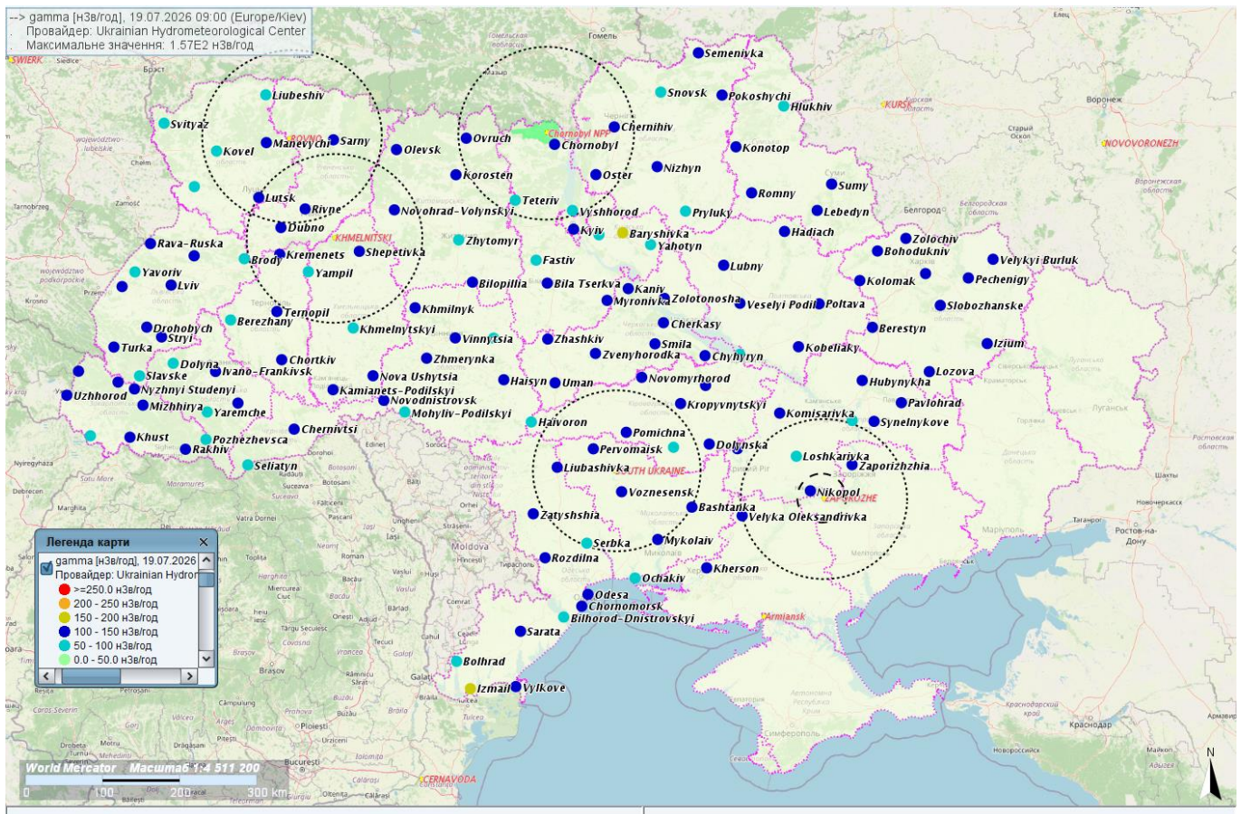
Рис1.Потужність дози Гамма-випромінювання на території України за результатами спостережень мережі НГМС станом на 09:00 (Київ) 19/07/2026.
