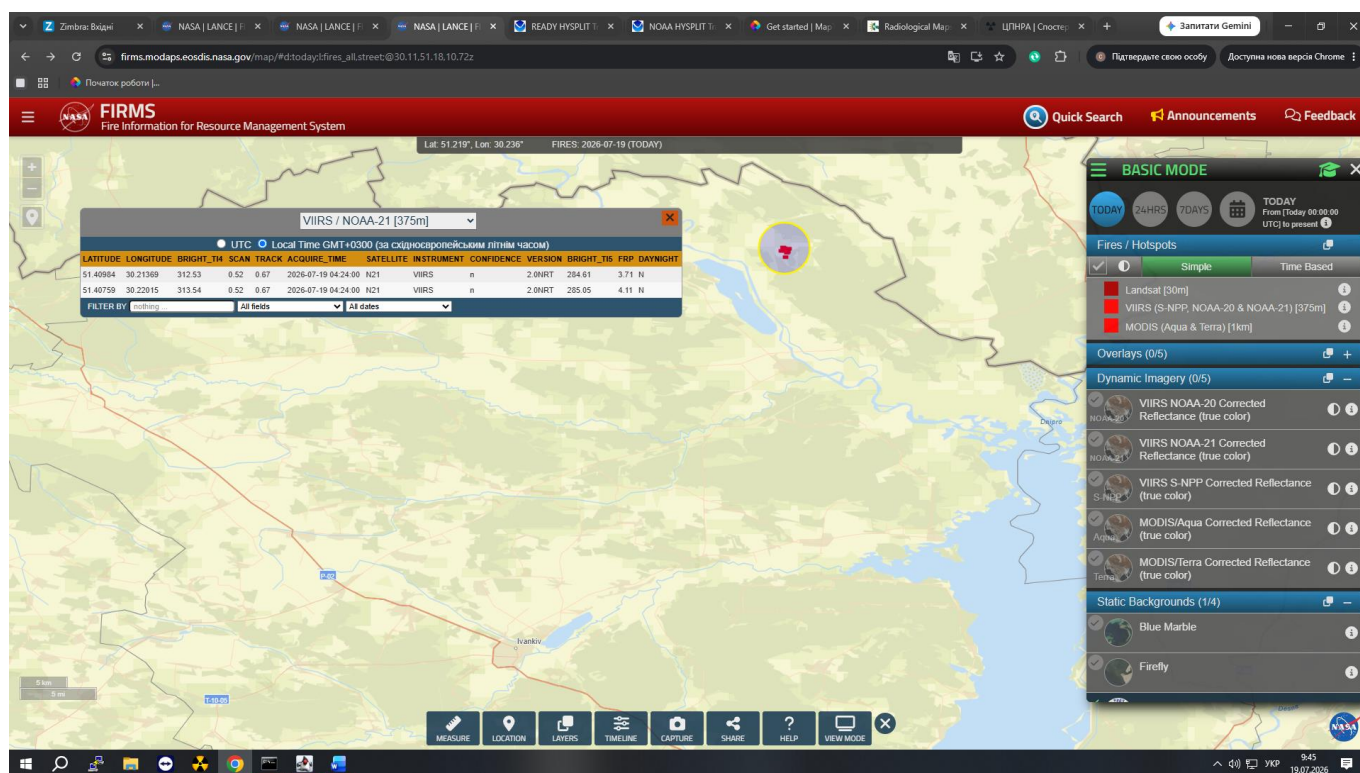
Рис.1.1 Карта-схема розташування осередків пожеж у ЗВ 19 липня 2026 року
