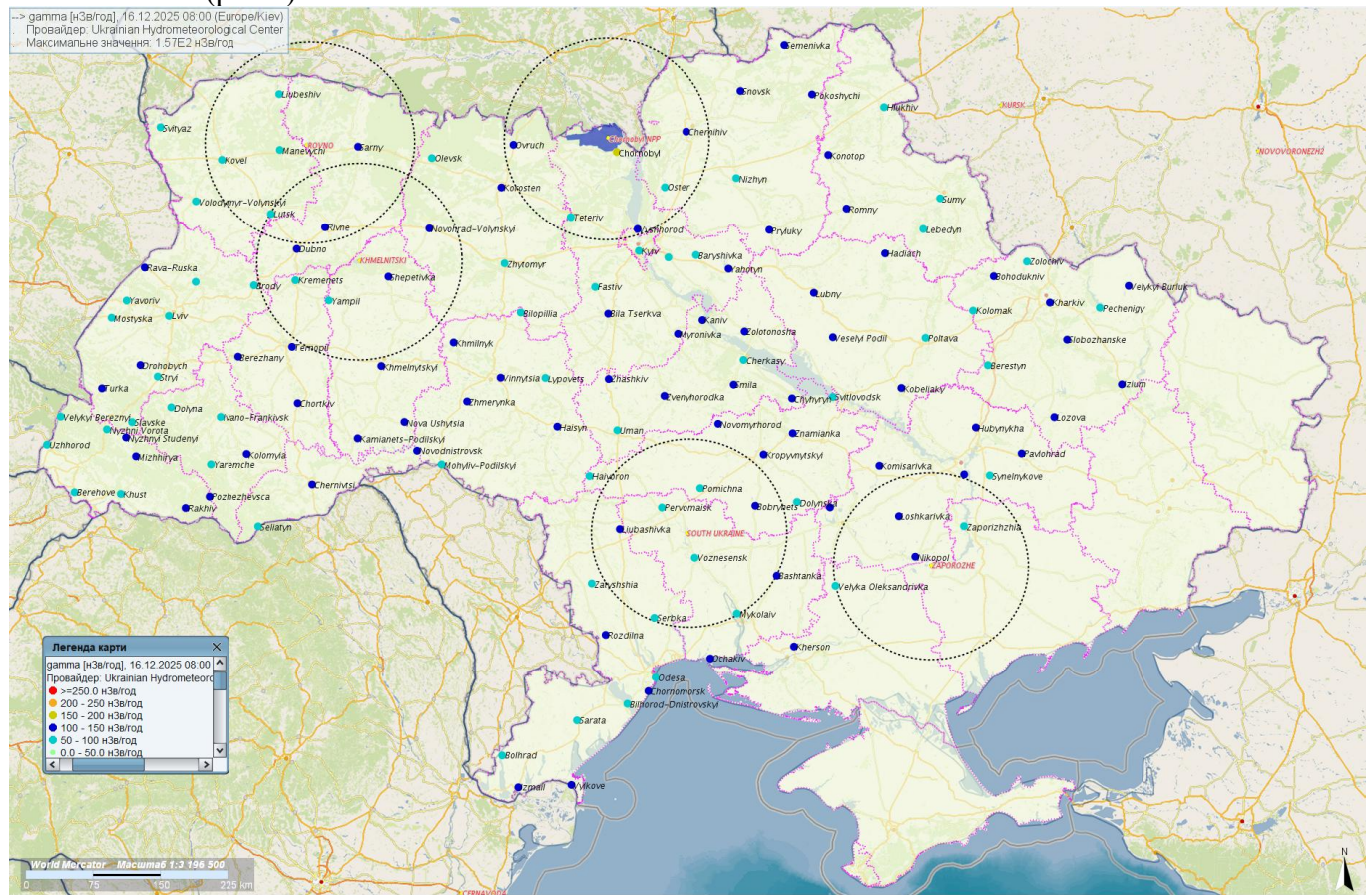
Рис1.Потужність дози Гамма-випромінювання на території України за результатами спостережень мережі НГМС станом на 08:00 (Київ) 16/12/2025.
