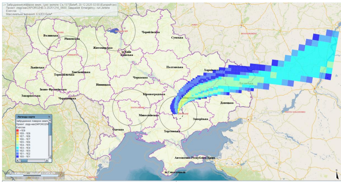
Рис.3. Результат моделювання просторового розподілу наслідків УРА на ЗАЕС (структура поля випадів довгоіснуючих радіоактивних елементів на прикладі Цезію-137). Щільність випадів представлено у Бк/м². Розрахунок умовного викиду ЗАЕС з 09:00 (Київ) 16/12/2025
