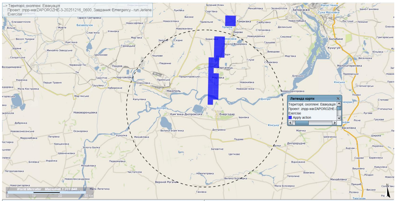
Рис.4. Результат моделювання просторового розподілу наслідків УРА на ЗАЕС (території, на яких рекомендована евакуація). Пунктиром позначено 30-ти кілометрову зону ЗАЕС. Розрахунок умовного викиду ЗАЕС з 09:00 (Київ) 16/12/2025
