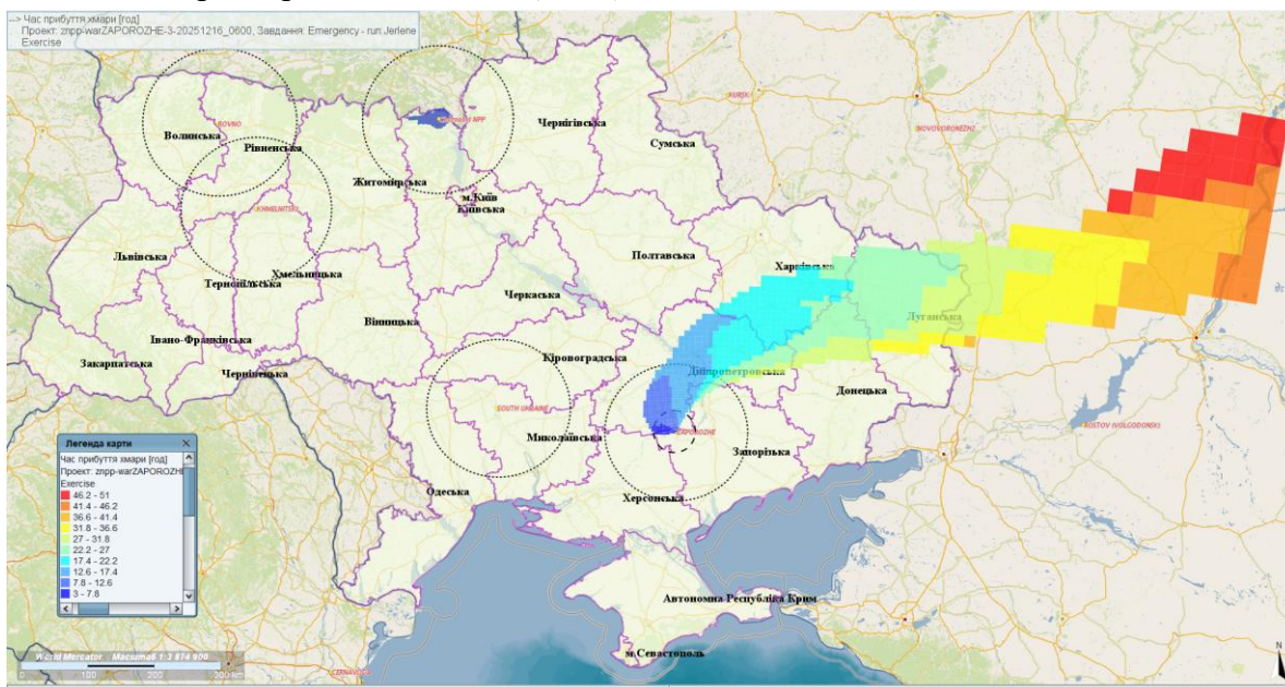
Рис.2. Прогноз поширення атмосферних мас з викидами ЗАЕС як наслідок УРА за 51 годину. Час прибуття хмари. Швидкість поширення забруднення у годинах. Розрахунок умовного викиду з 09:00 (Київ) 16/12/2025. Тривалість умовного викиду 24 год.
