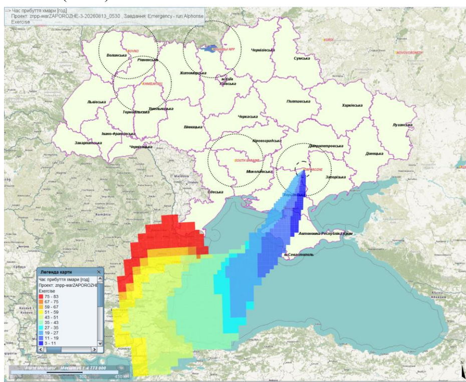
Рис.2. Прогноз поширення атмосферних мас з викидами ЗАЕС як наслідок УРА за 83 години. Час прибуття хмари. Швидкість поширення забруднення у годинах. Розрахунок умовного викиду з 08:30 (Київ) 13/08/2026. Тривалість умовного викиду 24 години.
