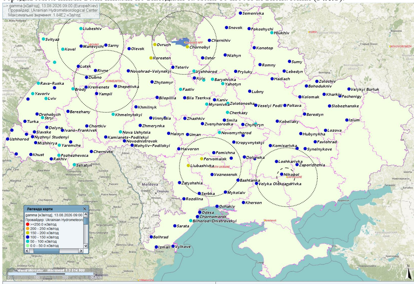
Рис.1. Потужність дози Гамма-випромінювання на території України за результатами спостережень мережі НГМС станом на 09:00 (Київ) 13/08/2026.
