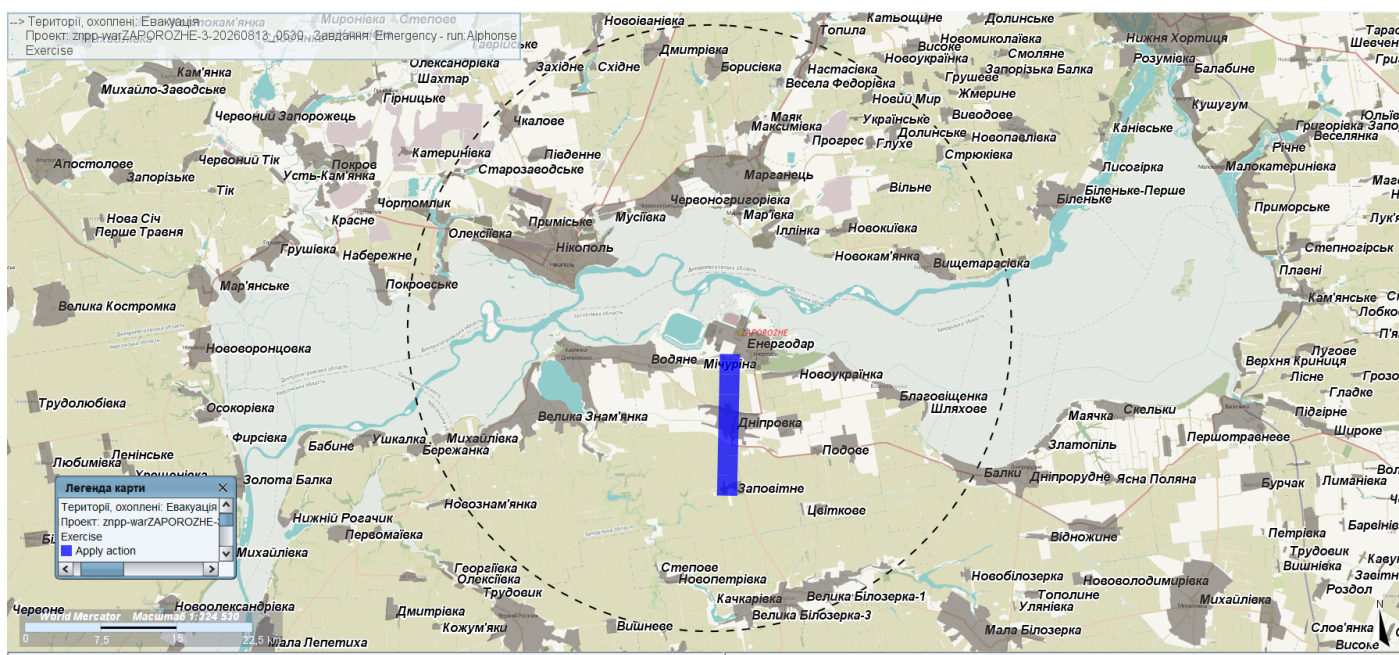
Рис.4. Результат моделювання просторового розподілу наслідків УРА на ЗАЕС (території, на яких рекомендована евакуація, згідно з НРБУ-97 таб. Д.8.1). Пунктиром позначено 30-ти кілометрову зону ЗАЕС. Розрахунок умовного викиду ЗАЕС з 08:30 (Київ) 13/08/2026
