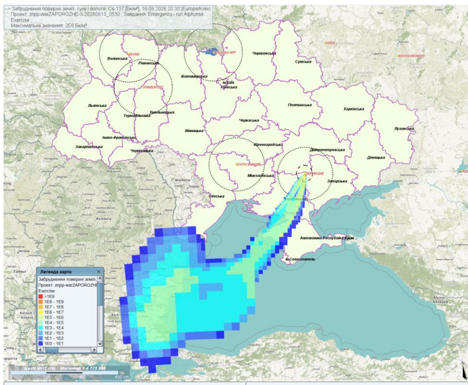
Рис.3. Результат моделювання просторового розподілу наслідків УРА на ЗАЕС (структура поля випадіння довгоіснуючих радіоактивних елементів на прикладі Цезію-137, згідно з НРБУ-97 таб. Д.8.1). Щільність випадіння представлено у Бк/м². Розрахунок умовного викиду ЗАЕС з 08:30 (Київ) 13/08/2026
