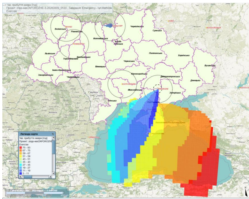
Рис.2. Прогноз поширення атмосферних мас з викидами ЗАЕС як наслідок УРА за 83 години. Час прибуття хмари. Швидкість поширення забруднення у годинах. Розрахунок умовного викиду з 08:30 (Київ) 09/08/2026. Тривалість умовного викиду 24 години.
