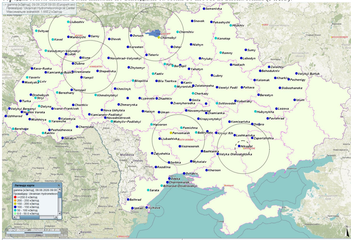
Рис.1. Потужність дози Гамма-випромінювання на території України за результатами спостережень мережі НГМС станом на 09:00 (Київ) 09/08/2026.
