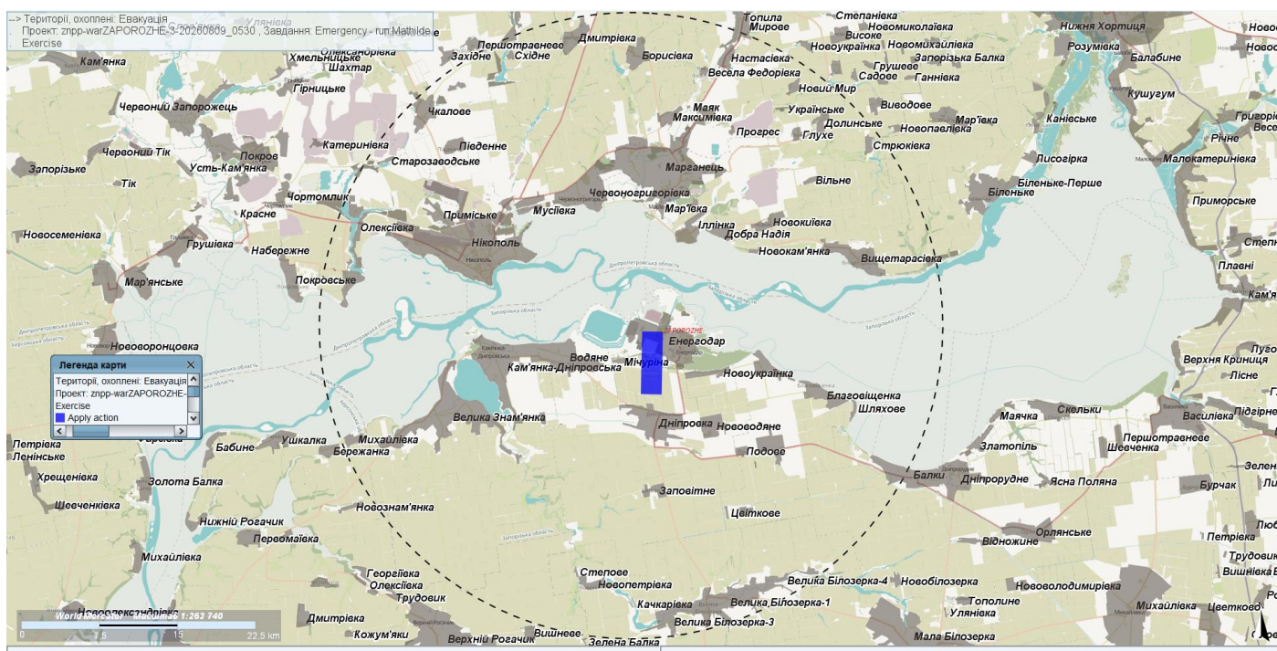
Рис.4. Результат моделювання просторового розподілу наслідків УРА на ЗАЕС (території, на яких рекомендована евакуація, згідно з НРБУ-97 таб. Д.8.1.). Пунктиром позначено 30-ти кілометрову зону ЗАЕС. Розрахунок умовного викиду ЗАЕС з 08:30 (Київ) 09/08/2026
