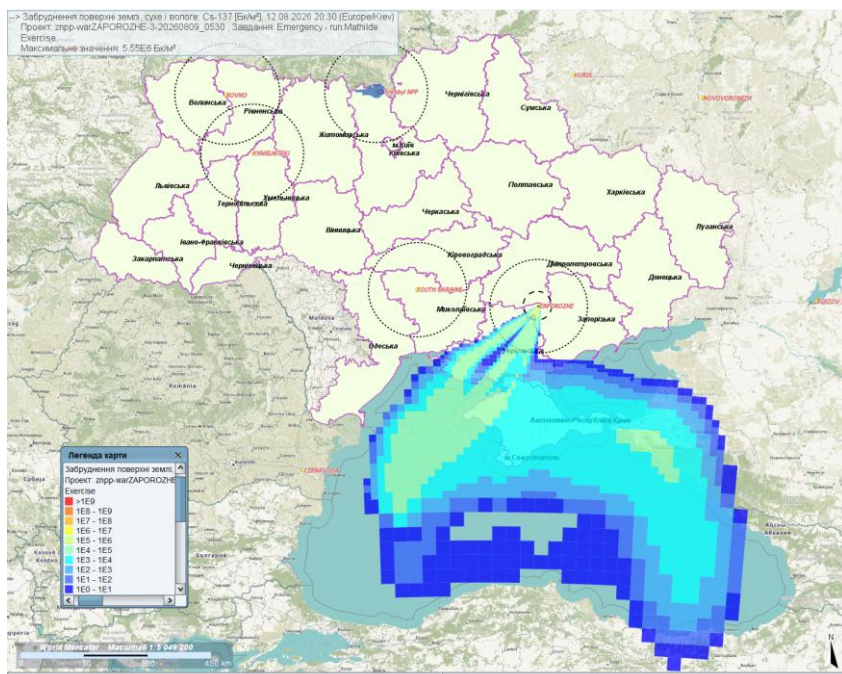
Рис.3. Результат моделювання просторового розподілу наслідків УРА на ЗАЕС (структура поля випадінь довгоіснуючих радіоактивних елементів на прикладі Цезію-137, згідно з НРБУ-97 таб. Д.8.1.). Щільність випадінь представлено у Бк/м². Розрахунок умовного викиду ЗАЕС з 08:30 (Київ) 09/08/2026
