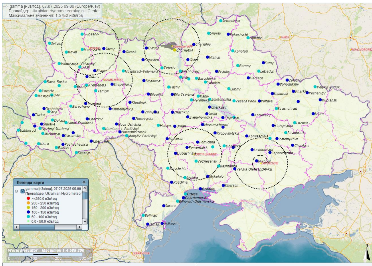
Рис.1.Потужність експозиційної дози на території України за результатами спостережень мережі НГМС станом на 09:00 (Київ) 07/07/2025.
