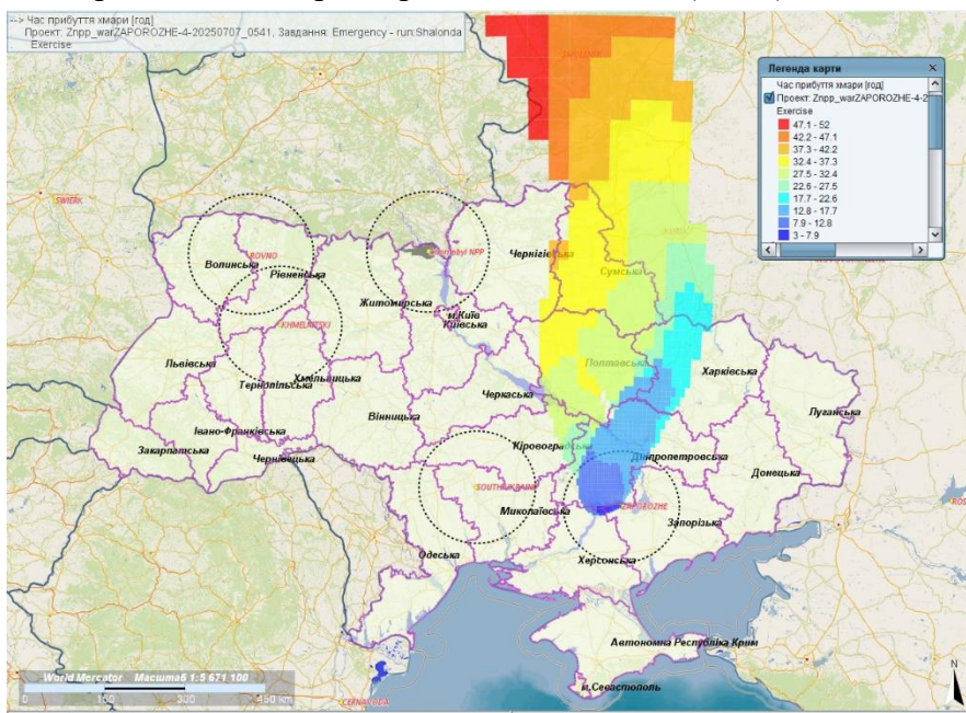
Рис.2. Прогноз поширення атмосферних мас з викидами ЗАЕС як наслідок УРА за 52 години. Час прибуття хмари. Швидкість поширення забруднення у годинах. Розрахунок умовного викиду з 09:00 (Київ) 07/07/2025. Тривалість умовного викиду 24 год.
