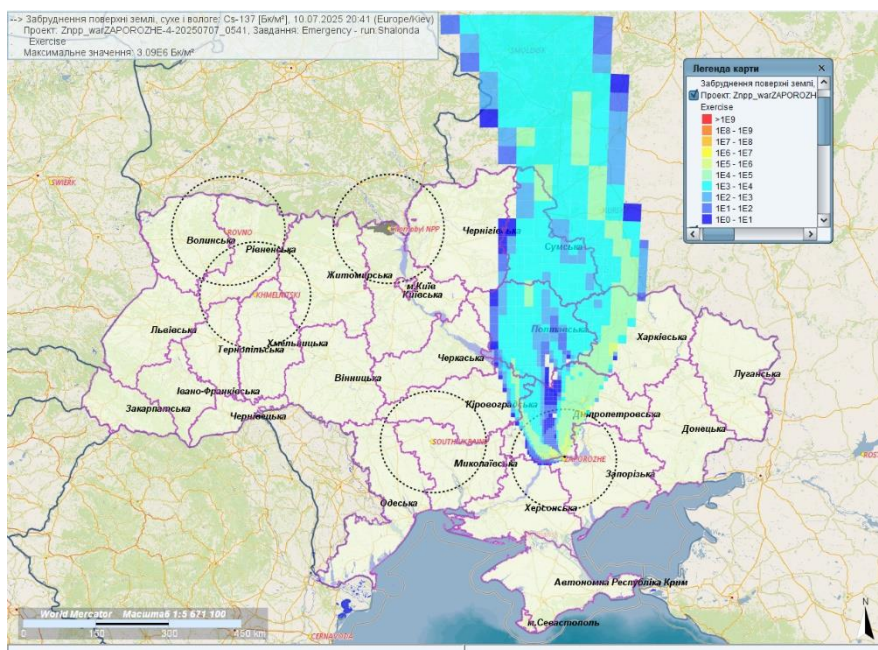
Рис.3. Результат моделювання просторового розподілу наслідків УРА на ЗАЕС (структура поля випадіннь довгоіснуючих радіоактивних елементів на прикладі Цезію-137). Щільність випадіннь представлено у Бк/м2. Розрахунок умовного викиду ЗАЕС з 09:00 (Київ) 07/07/2025
