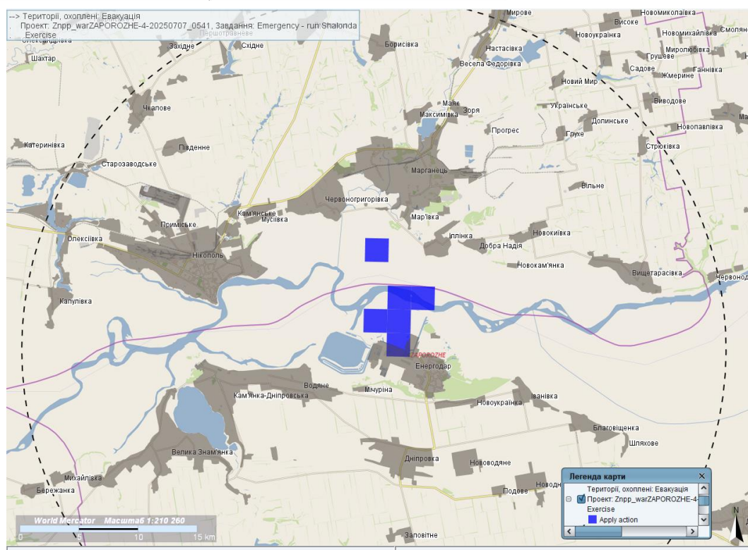
Рис.4. Результат моделювання просторового розподілу наслідків УРА на ЗАЕС (території, на яких рекомендована евакуація). Пунктиром позначено 30-кілометрову зону ЗАЕС. Розрахунок умовного викиду ЗАЕС з 09:00 (Київ) 07/07/2025
