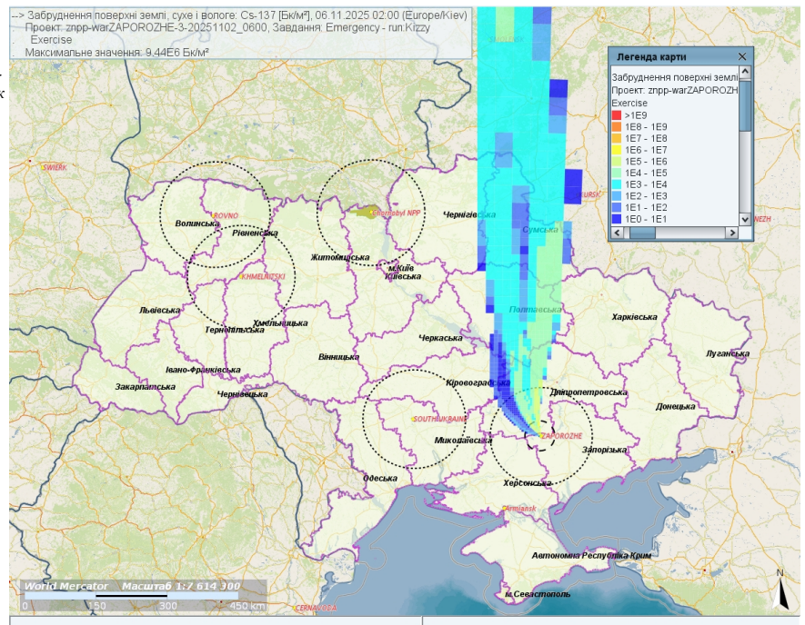
Рис.3. Результат моделювання просторового розподілу наслідків УРА на ЗАЕС (структура поля випадінь довгоіснуючих радіоактивних елементів на прикладі Цезію-137). Щільність випадінь представлено у Бк/м². Розрахунок умовного викиду ЗАЕС з 09:00 (Київ) 02/11/2025
