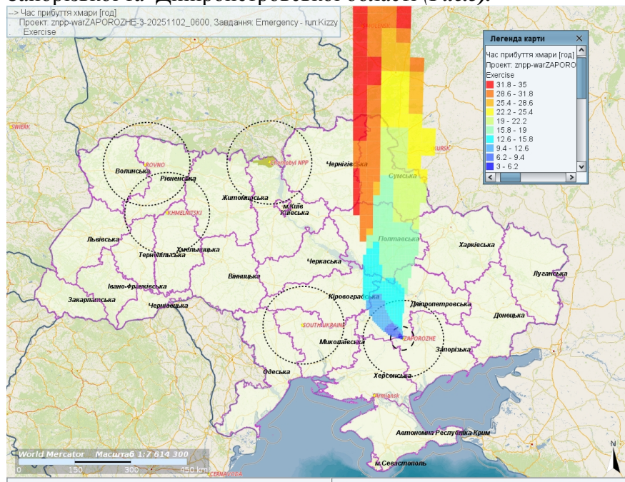
Рис.2. Прогноз поширення атмосферних мас з викидами ЗАЕС як наслідок УРА за 35 годин. Час прибуття хмари. Швидкість поширення забруднення у годинах. Розрахунок умовного викиду з 09:00 (Київ) 02/11/2025. Тривалість умовного викиду 24 год.
