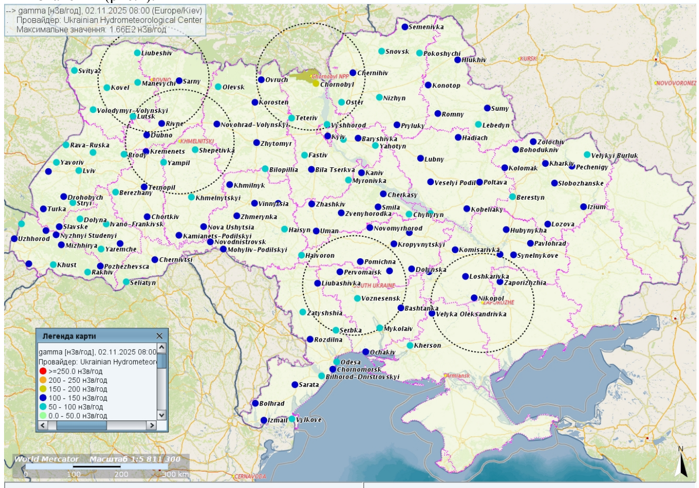
Рис.1.Потужність дози Гамма-випромінювання на території України за результатами спостережень мережі НГМС станом на 08:00 (Київ) 02/11/2025.
