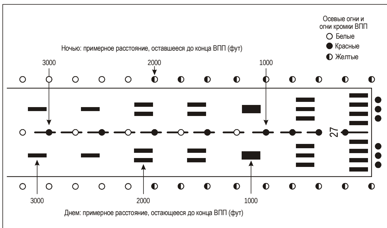
Рис. 4-16. Маркировка и огни ВПП, оборудованной для точного захода на посадку согласно стандартам ИКАО/ФАУ (Учебное пособие ФАУ по сдвигу ветра, 1987 г., адаптировано ИКАО.)
