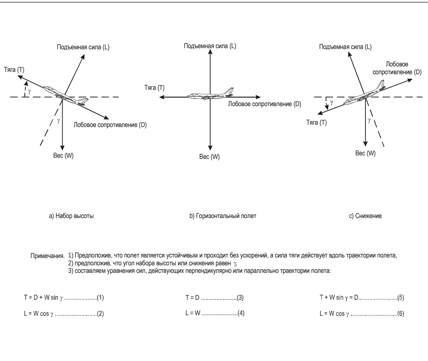
Рис. 4-1. Силы, действующие на воздушное судно в полете
