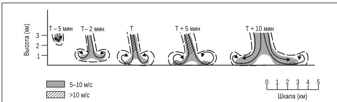
Рис. 3-17. Вертикальный разрез развития поля ветра, относящегося к микропорыву; T- время начальной дивергенции у земной поверхности. Штриховкой обозначены векторные скорости (Вильсон, Робертс, Кессинджер и Маккарти, 1984 г.)
