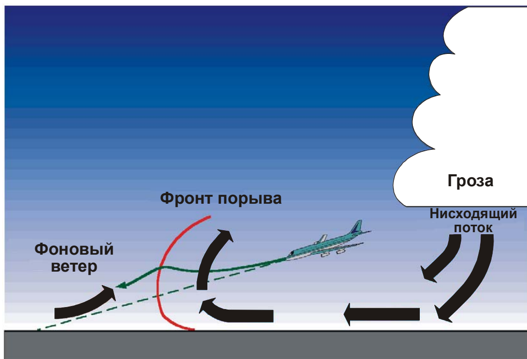
Рис. А4-4. Сдвиг ветра, вызванный фронтом порывов
