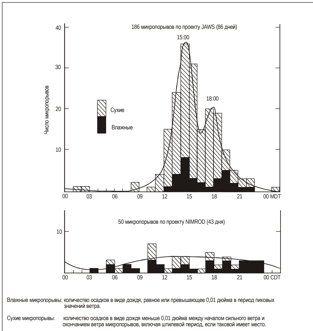
Рис. 3-13. Суточные изменения приземных микропорывов всех степеней интенсивности, измеренные на 27 станциях РАМ (Фудзита и Вакимото, 1983 г., адаптировано ИКАО)
