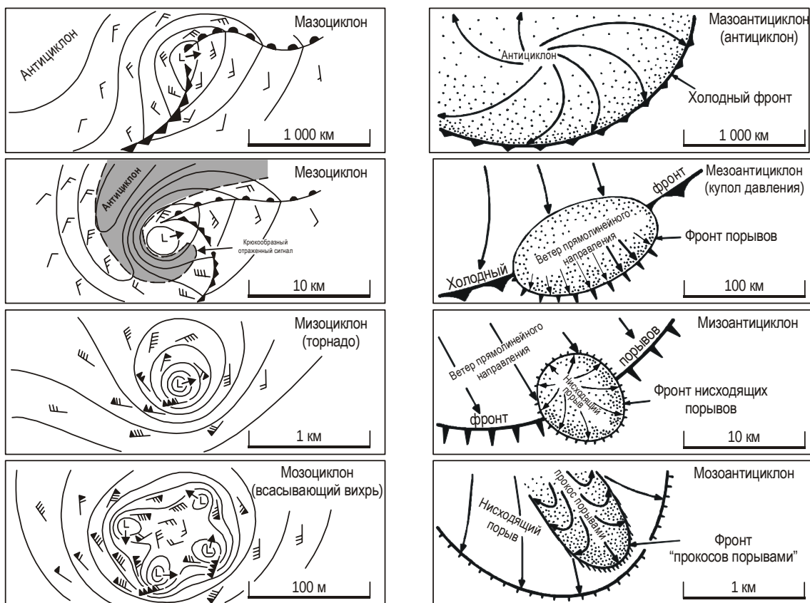
а) Мазо-, мезо-, мизо- и мозоциклоны в контексте обобщенных планетарных масштабов. Последовательность соответствует порядку расположения гласных а, е, и, о и у.
