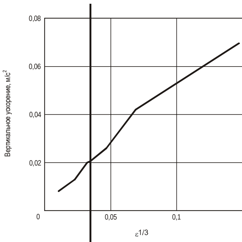
Рис. 5-6. Изменение вертикального ускорения относительно кубического корня скорости затухания вихря (Сорейд, Боуг, Эхернбергер, Ханнон и Боудл, 2000 г.)
