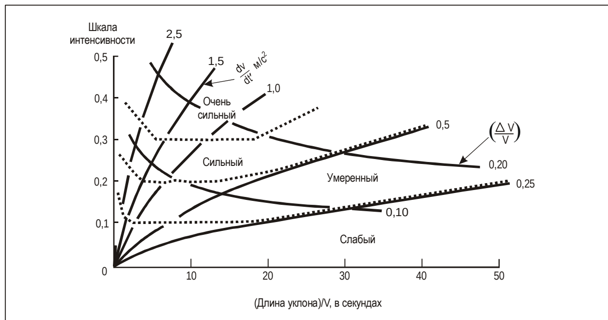
Рис. 5-7. Предлагаемая форма граничных значений интенсивности (Вудфилд и Вудс, 1984 г.)
