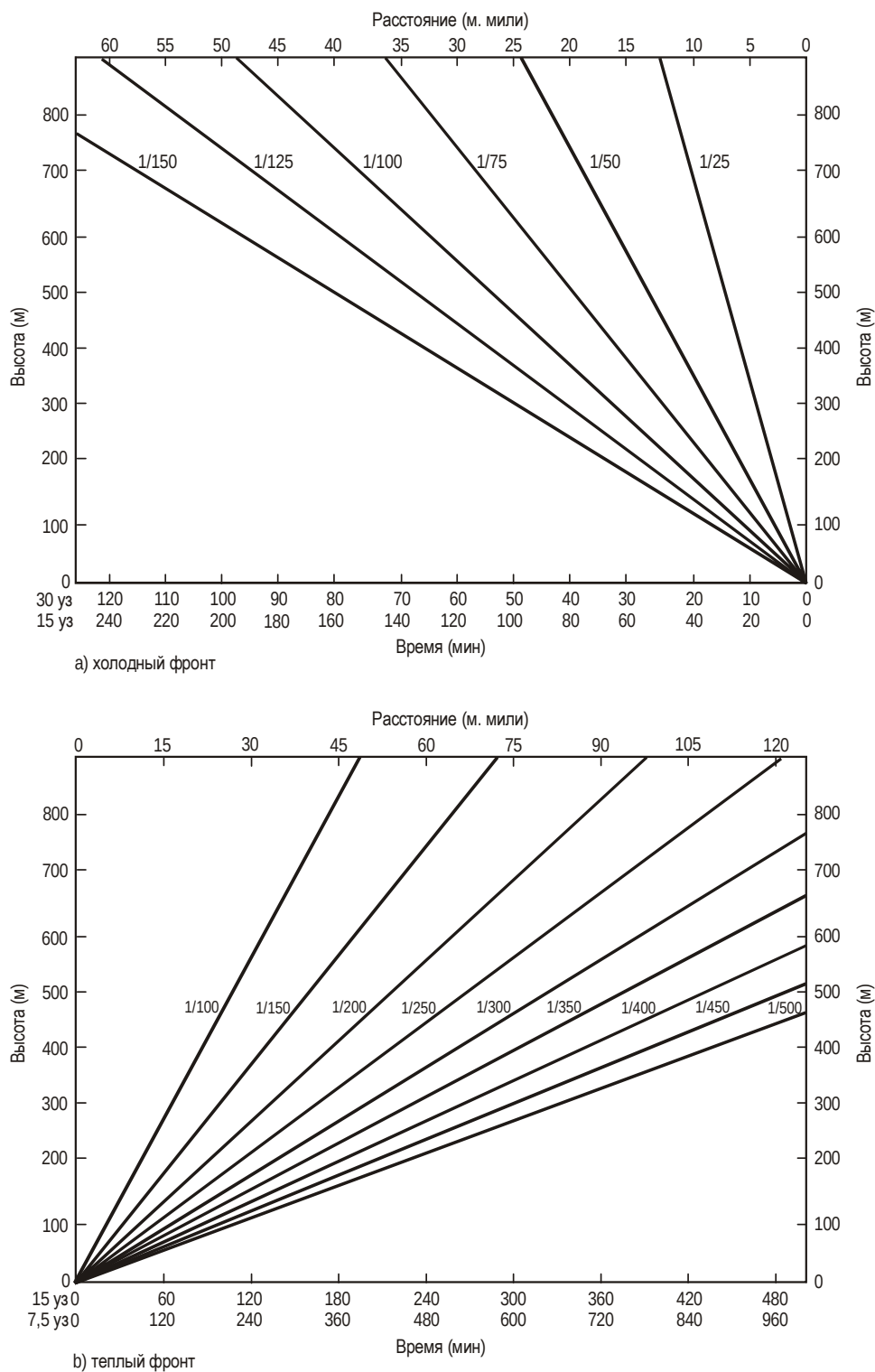
Рис. 5-8. Высота теплого и холодного фронтов в соотношении с расстоянием/временем до аэропорта при различных наклонах (Баднер, 1979 г., адаптировано ИКАО)
