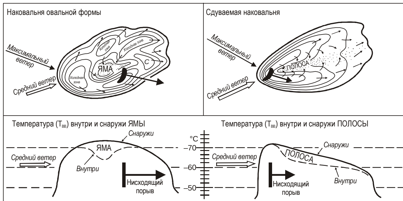
Рис. 5-15. Схематические диаграммы в плане и профиле распределения температуры на вершине облака ( T_{vv} ). Средний ветер означает ветер среднего слоя от 0 до 3 км или от 3 до 6 км ниже высоты максимального ветра вблизи уровня наковальни. Основано на результатах инфракрасного анализа четырех случаев нисходящих порывов (Фудзита, 1978 г., адаптировано ИКАО)
