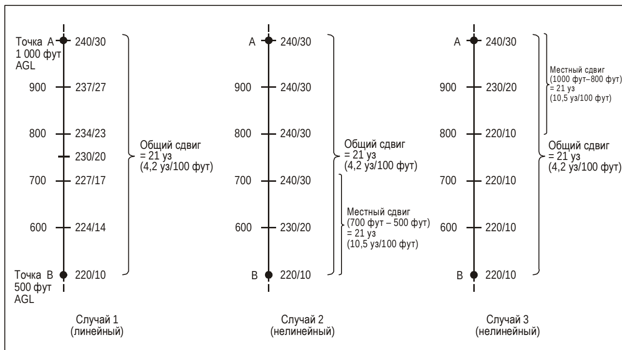
Рис. 2-3. Линейный и нелинейный сдвиг ветра
