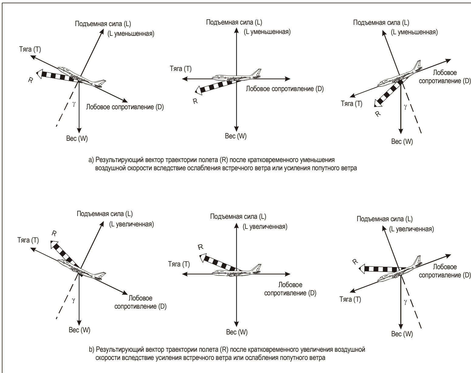
Рис. 4-2. Результирующий вектор траектории полета, связанный со сдвигом горизонтального ветра
