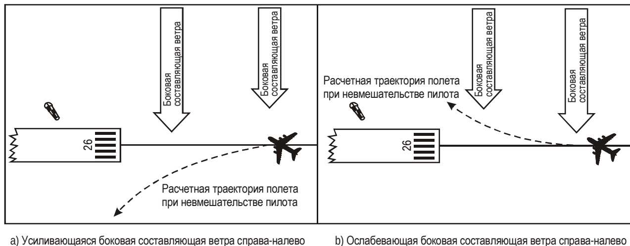
Рис. 4-9. Воздействие сдвига бокового ветра на воздушное судно при предполагаемом невмешательстве пилота
