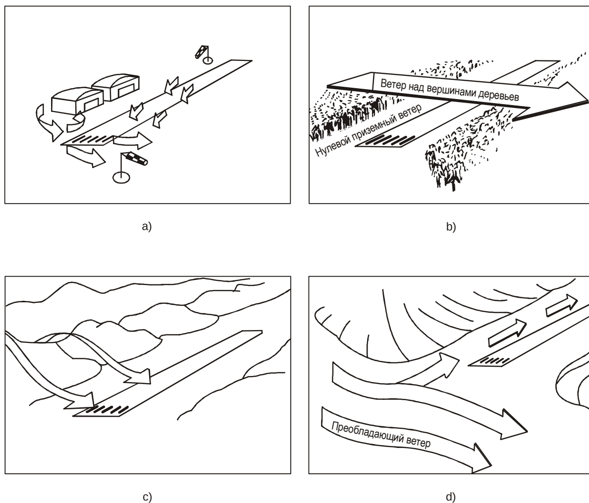
Рис. 3-3. Ветер, обтекающий препятствия
