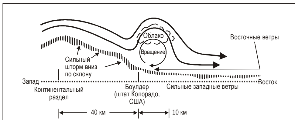
Рис. 5-11. Схематический вертикальный разрез, проходящий через Боулдер (штат Колорадо, Соединенные Штаты Америки) на 24 января 1982 г., предположительно репрезентативный в отношении поля среднего потока, по состоянию на 09.00–18.00 по среднему солнечному времени. Хотя в зоне вокруг Боулдера преобладали ветры общего направления, на высоте 2-3 км над уровнем земли в смолисто-кучево-облачности, систематически образующейся к западу от Боулдера, наблюдались сильные западные ветры (Зипсер и Бедард, 1982 г., адаптировано ИКАО)
