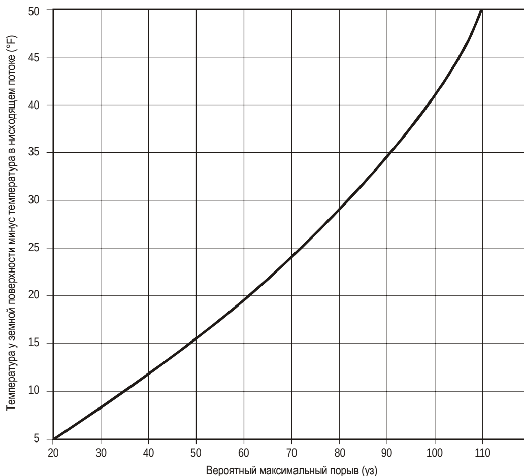
Рис. 5-12. Эмпирические прогнозы вероятных максимальных порывов (Джорж, 1960 г.)
