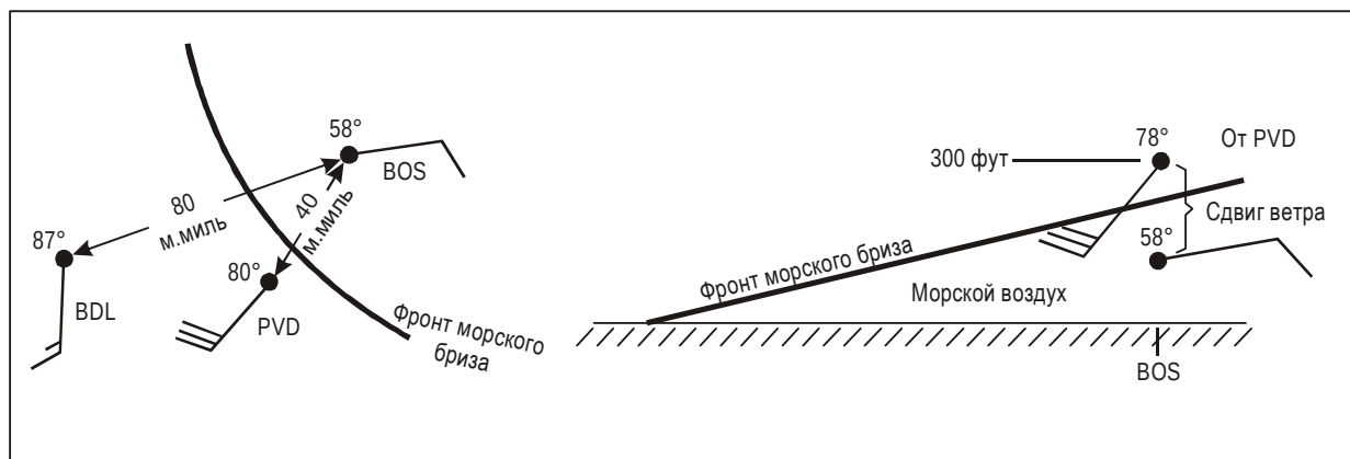
Рис. 5-9. Сдвиг ветра, связанный с морским бризом (Баднер, 1979 г.)
