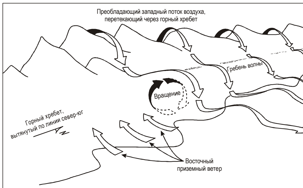
Рис. 3-4. Подветренные волны
